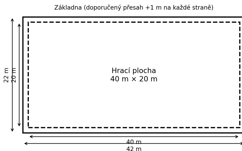
Obrázek 3: Schéma základních rozměrů FIFA ARÉNY (orientační; závazné parametry stanoví technické přílohy).
